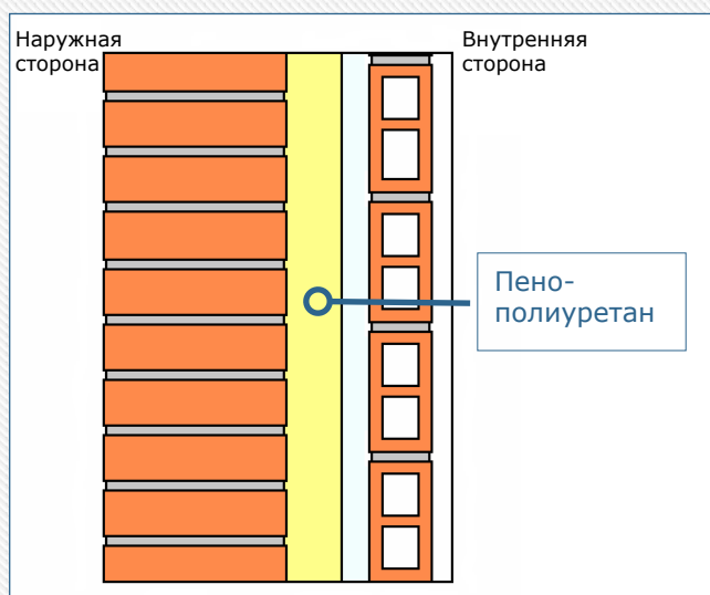
Рисунок 3: Стандартное конструктивное решение в Испании
