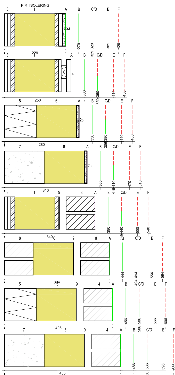
Figur 3: Nybyggeri, ydervægskonstruktioner
